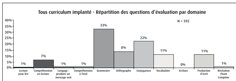
Graphique 2.1.2 : Curriculums implantés : répartition par domaine en français dans cinq pays (apprentissages formels et non formels)
