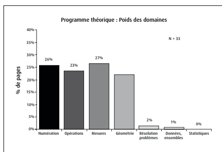
Graphique 2.1.3 : Curriculums officiels : répartition par domaine en mathématiques dans cinq pays
