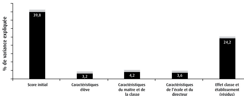
Graphique 4.5 : Modèle de production scolaire PASEC
