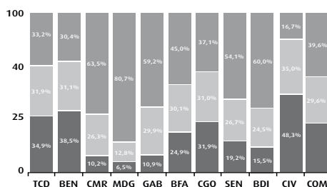
Mathématiques - fin de 5 e année
